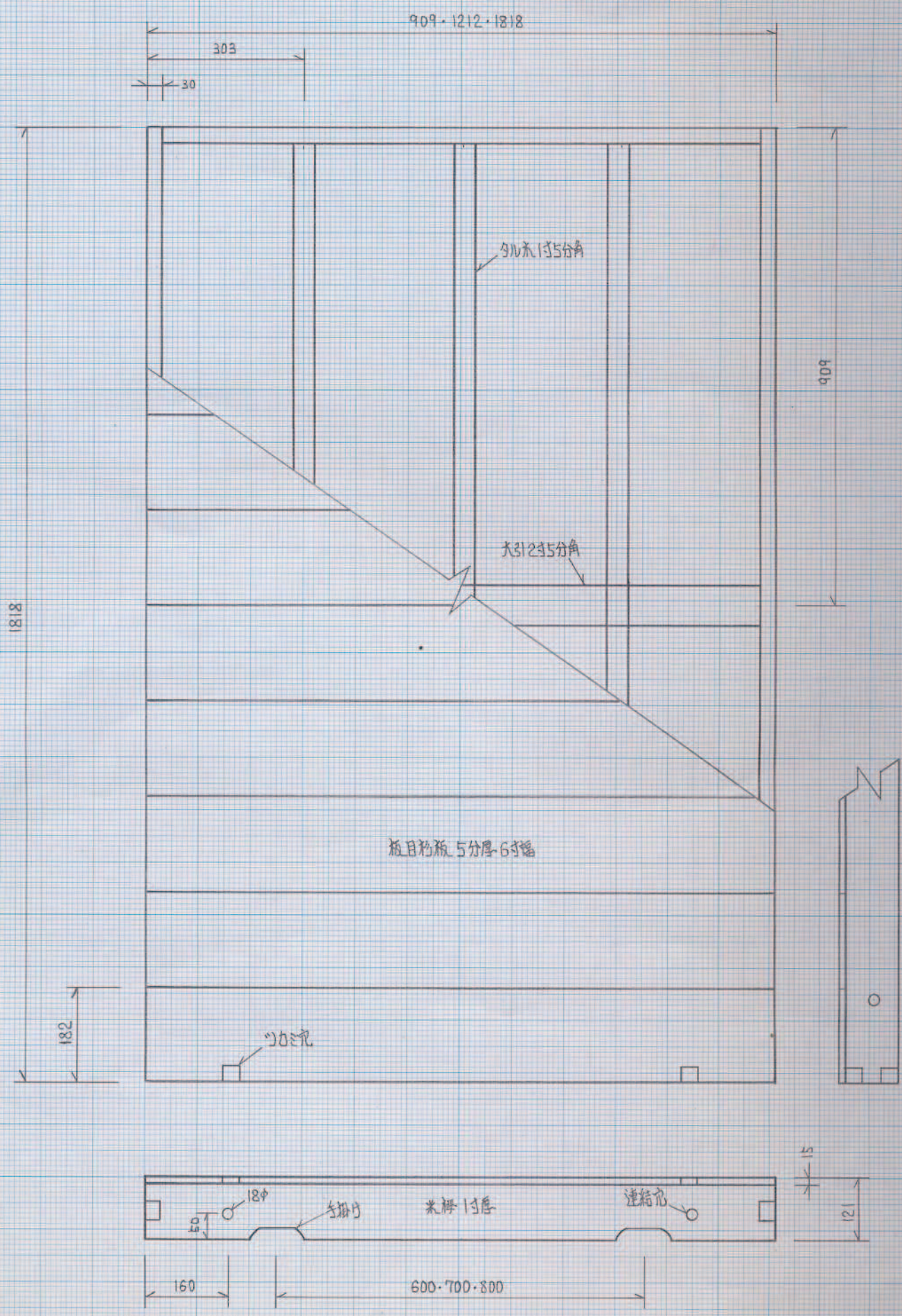
市民会館舞台平台仕様 1/10
