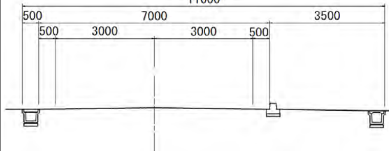
標準断面図 11000
