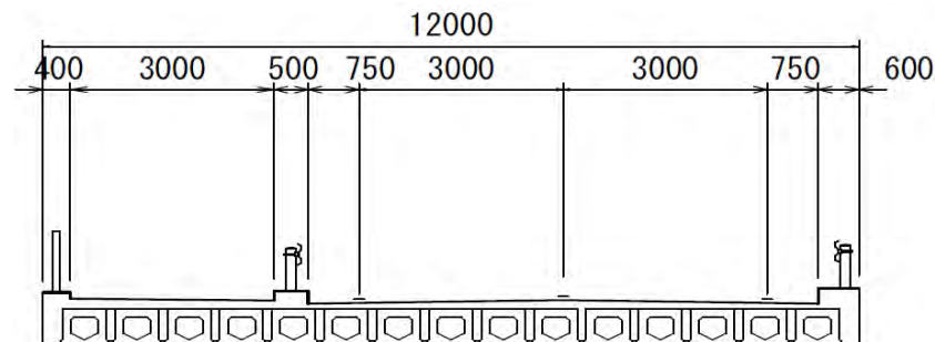
通学橋断面図
