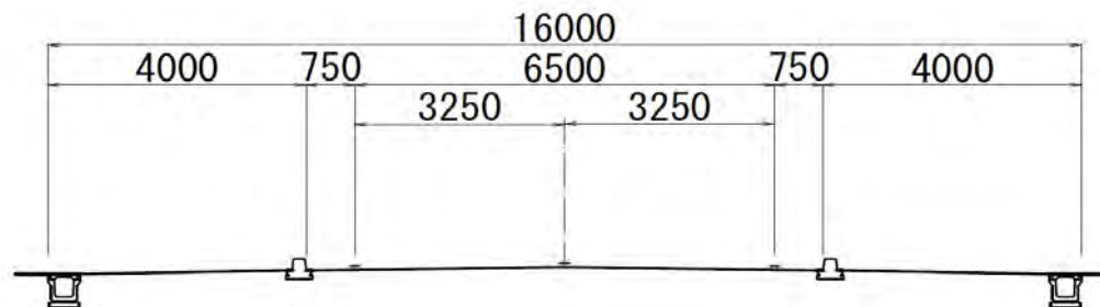
標準断面図
