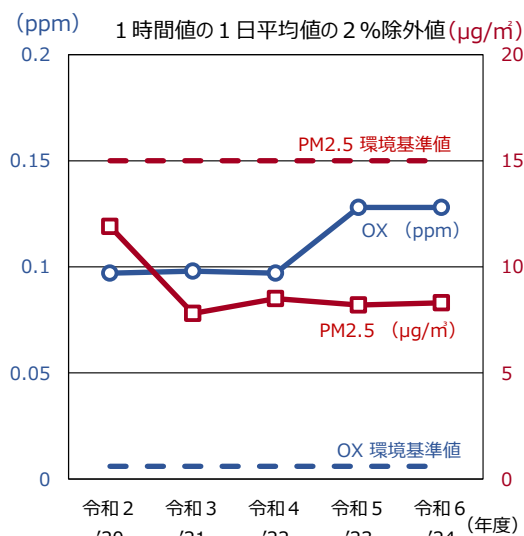
[O x 、PM2.5]
