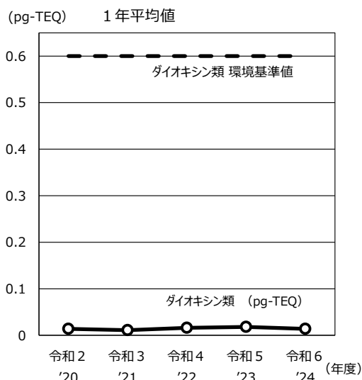
[ダイオキシン類]
