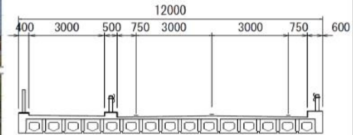
通学橋 断面図
