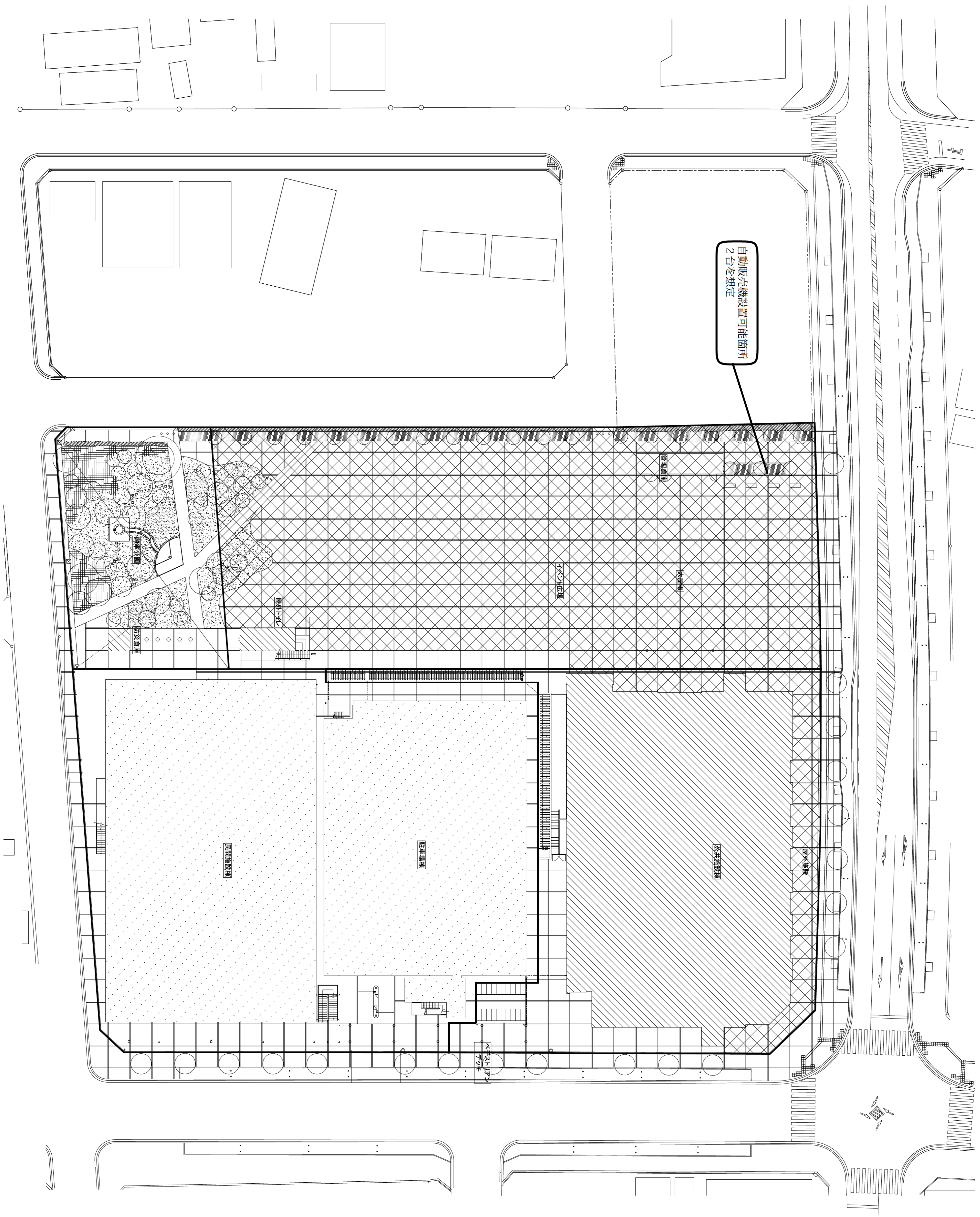
配置図 A1=1:300 A3=1:600
