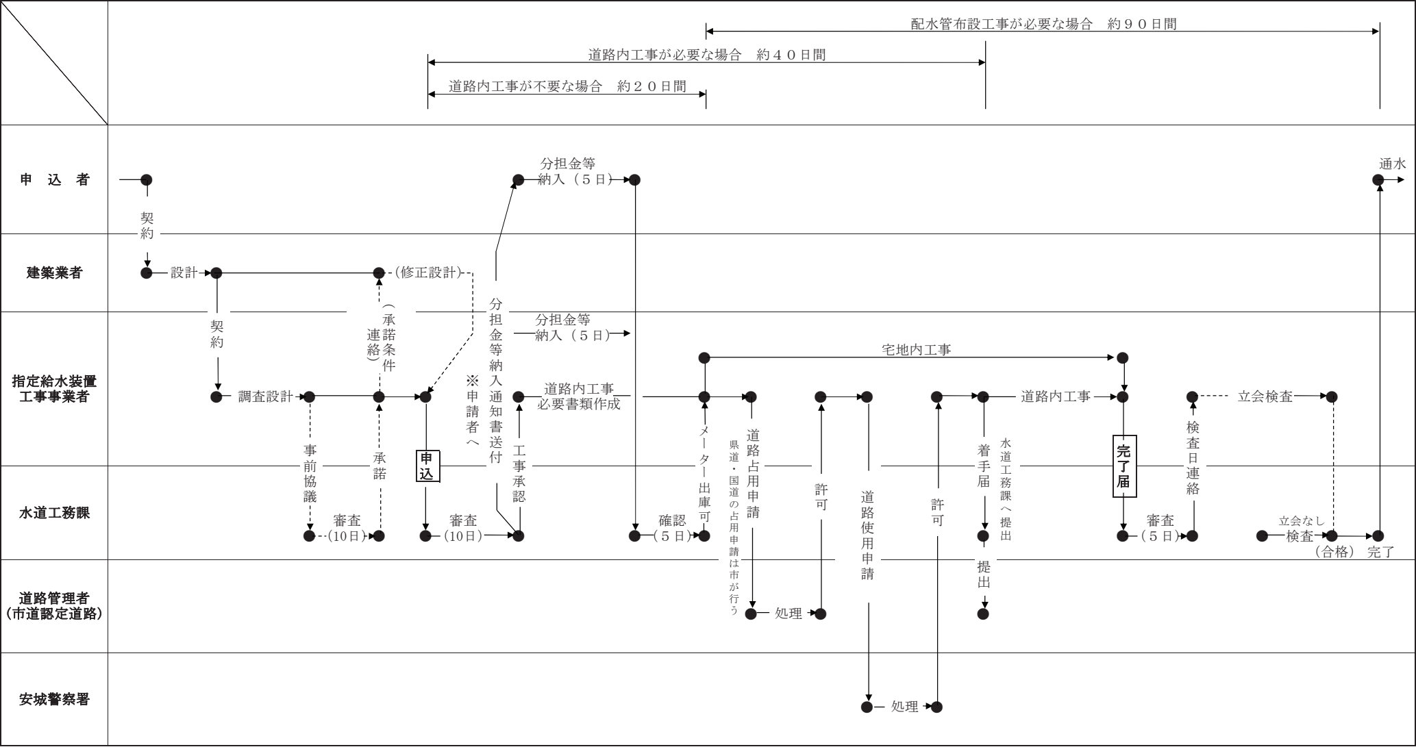
給水装置の工事申込から施工までのフロー図（標準）
