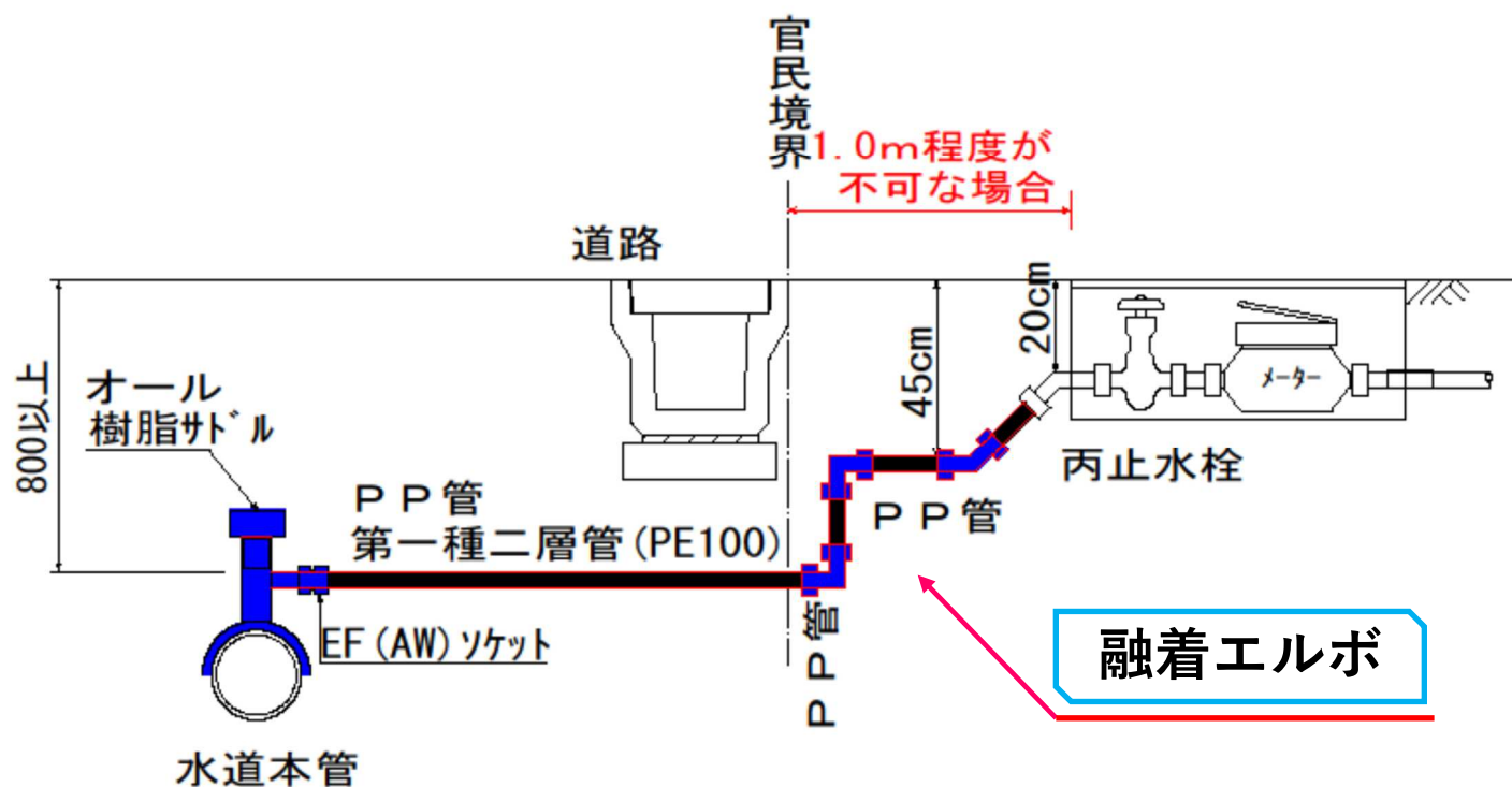
給水管参考図
