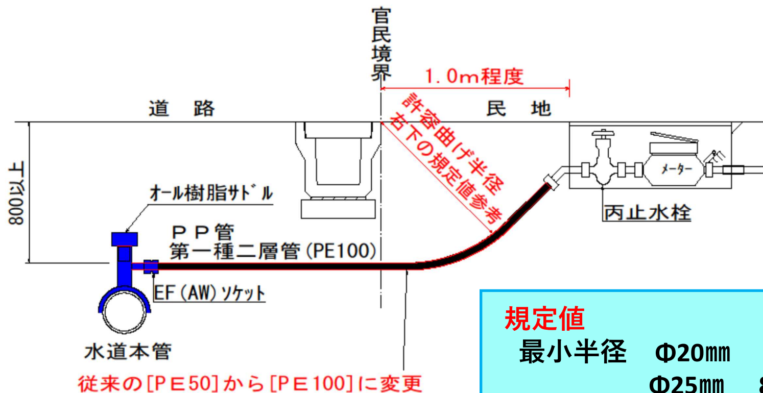
給水管参考図
