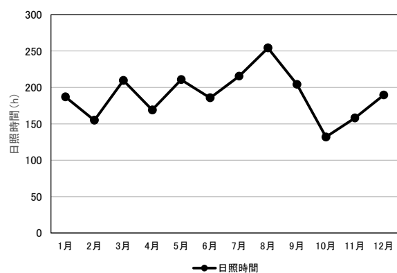
図 4.1-2 大府地域気象観測所における気象概況（令和6年）
