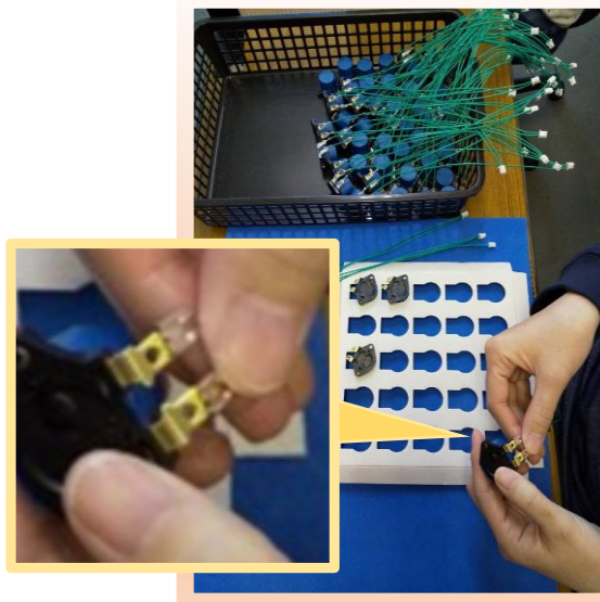
ファンヒーター用リード線組み立てです。差し込む方向を間違えない様の一つずつ丁寧に行っています。
