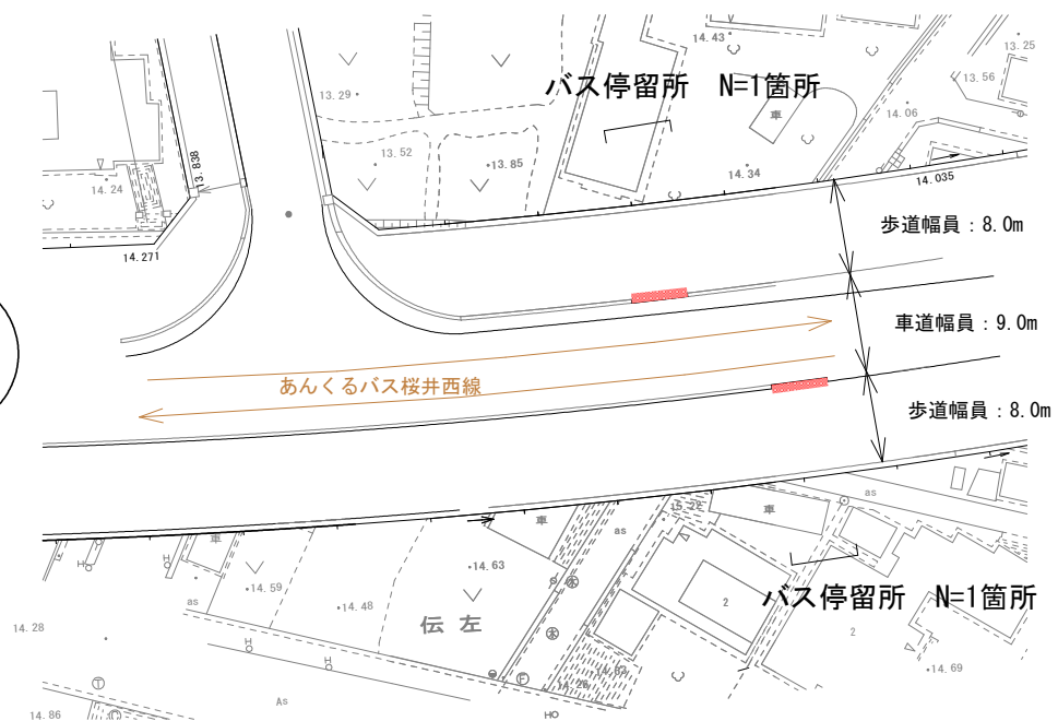
平面図 S=1/500
