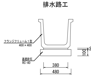
構造図 S=1:20
