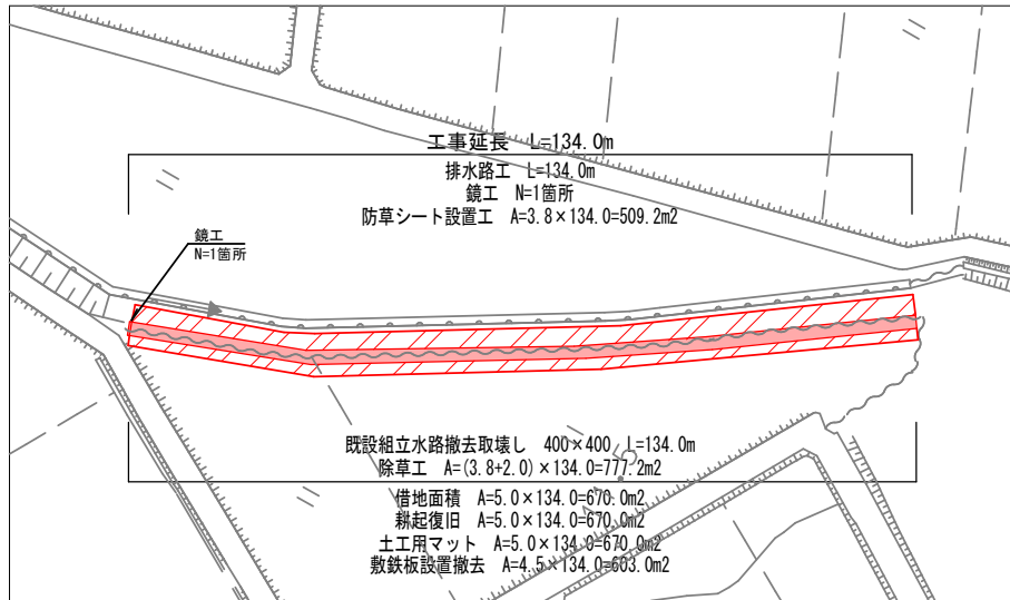
平面図 S=1:1000
